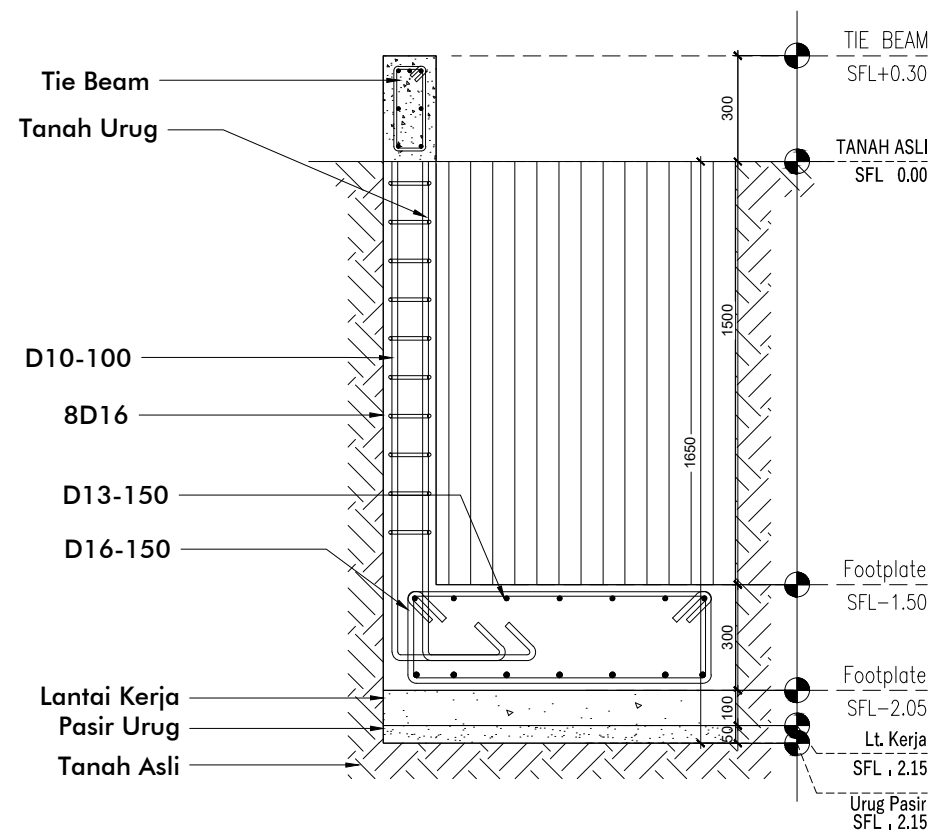
2 STR POTONGAN A 1: 20
