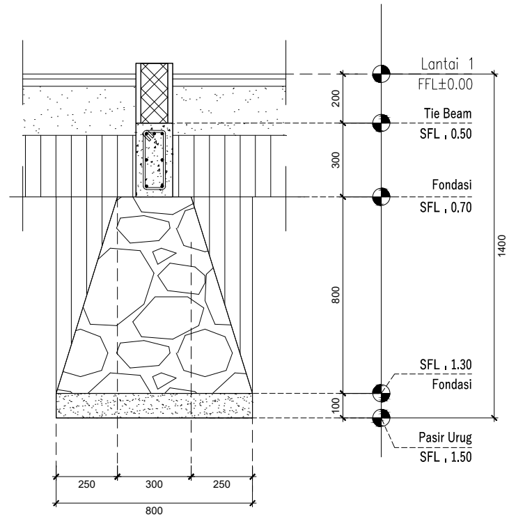
2 STR POTONGAN a-a 1: 20
