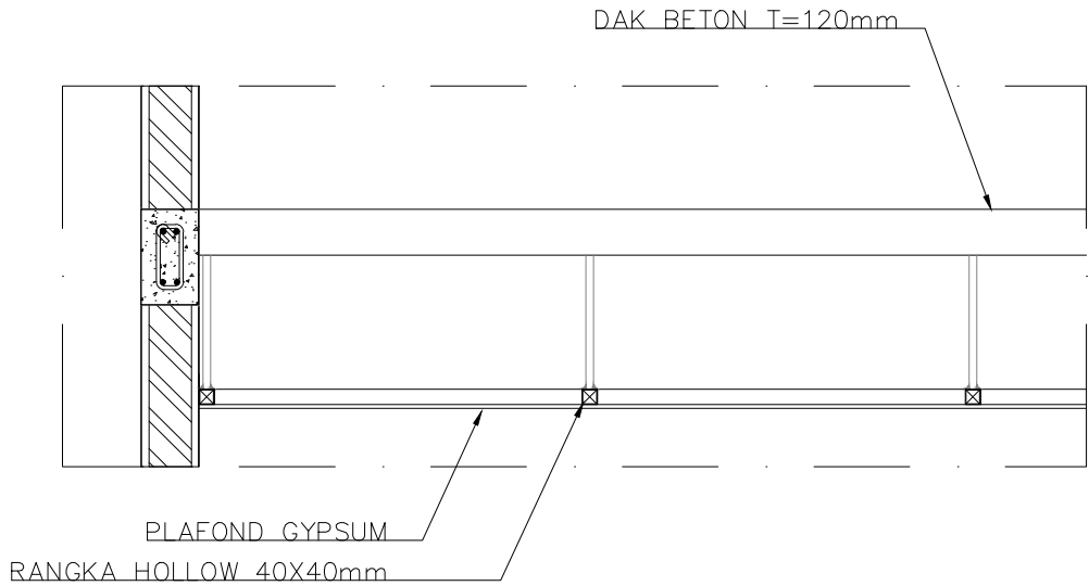
CL ARS POTONGAN D-D 1:15
