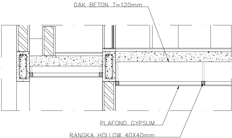
CL ARS POTONGAN A-A 1:15
