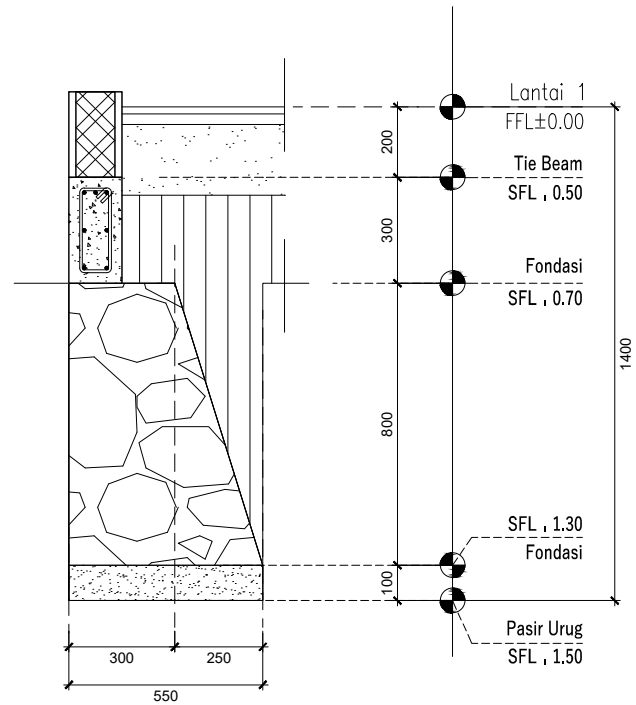
2 STR POTONGAN b-b 1: 20
