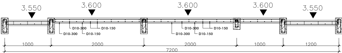
2 STR POTONGAN A-A 1: 30
