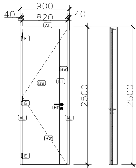
29 ARS TAMPAK DEPAN P1 1:30
