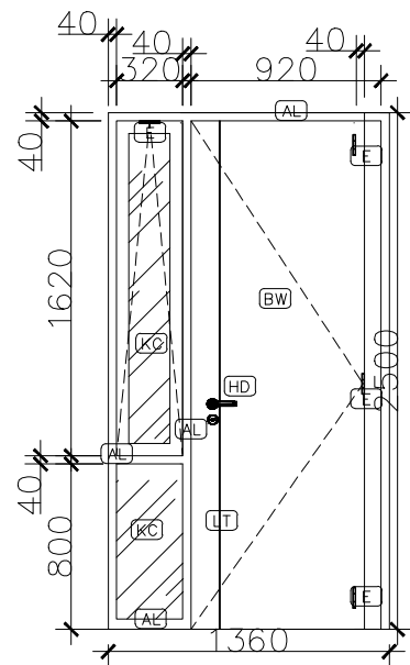
28 ARS TAMPAK DEPAN PJ1 1:30
