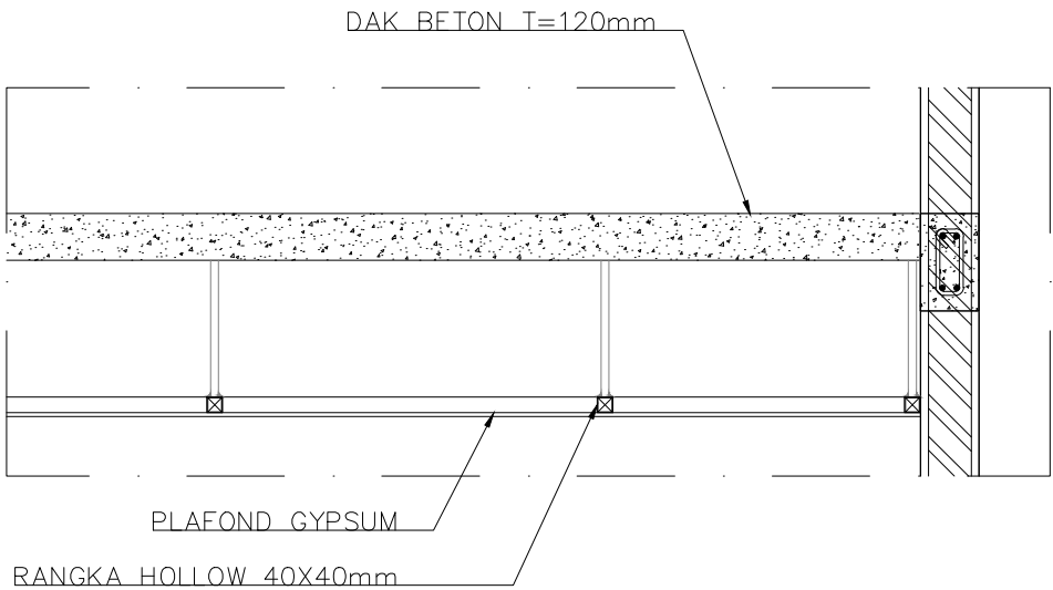
CL ARS POTONGAN C-C 1:15
