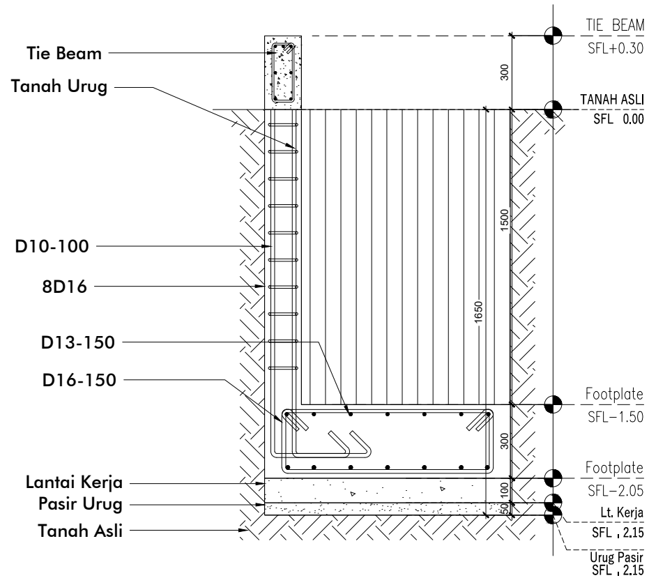
2 STR POTONGAN A 1: 20
